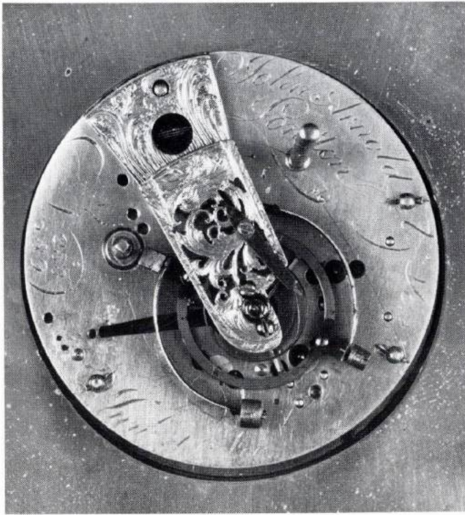
3 △ 3 John Arnolds Taschenuhr mit Chronometerhemmung von 1782. Die Unruh hat Wendelfeder und aufgeschraubte bimetallische Streifen für die Temperaturkompensation. Reguliert wird mit den Gewichtsschrauben am Unruhreif
