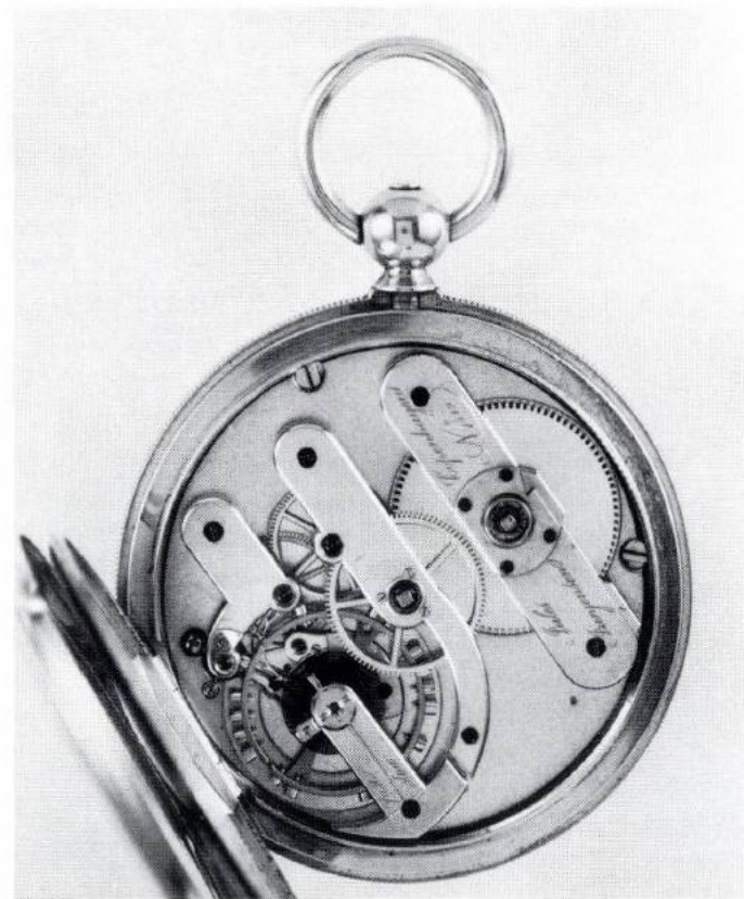
26 Taschenuhr mit Wippen-Chronometerhemmung, auf der Federhausbrücke signiert »Jules Jürgensen Copenhagen No. 7412«. Die Unruh hat Breguet-Spirale und Rückerzeiger
