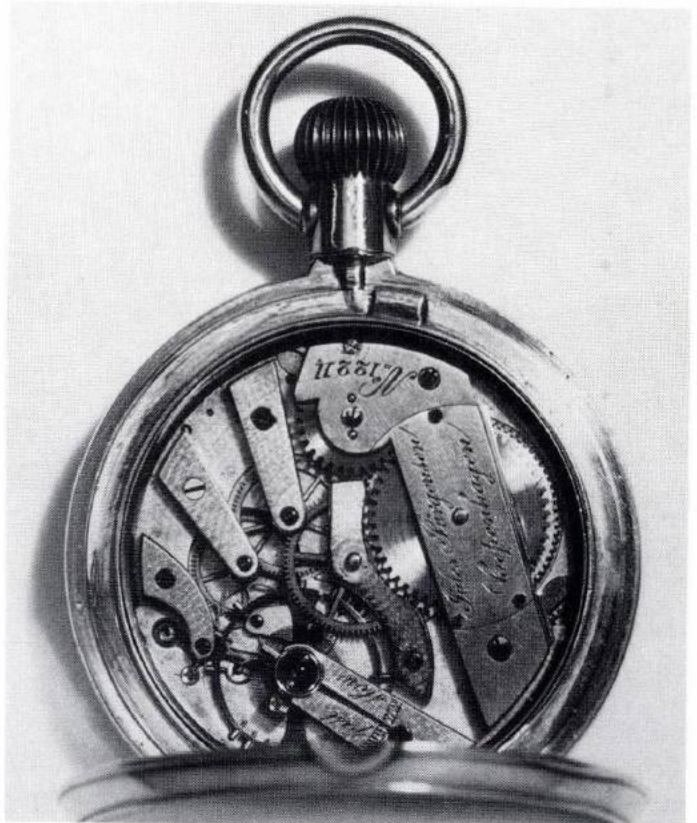
28 Taschenuhr mit Wippen-Chronometerhemmung und Remontoir-Aufzug, signiert »Jules Jürgensen Copenhagen No. 12211«. Die Gangpartie wurde gegenüber Abb. 26 nicht verändert, jedoch die Kloben und Brücken sind anders gestaltet
