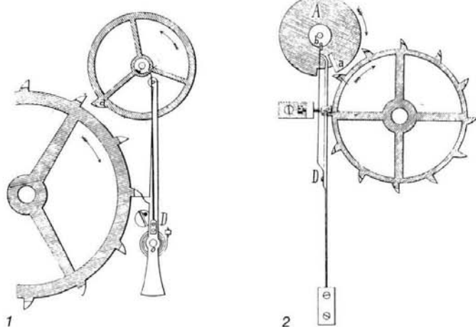
1 Die erste ab 1770 angewandte Chronometerhemmung mit Wippe für Seechronometer von John Arnold
