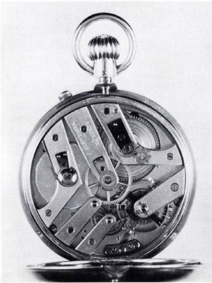
19 Der gut durchdachte Werkaufbau mit Kloben und Brücken läßt die Eingriffe der Zahnräder und die Chronometerhemmung mit Feder nach Earnshaw klar erkennen. Um das Werk flacher zu gestalten, wurde eine freischwingende Breguet-Spirale verwendet
