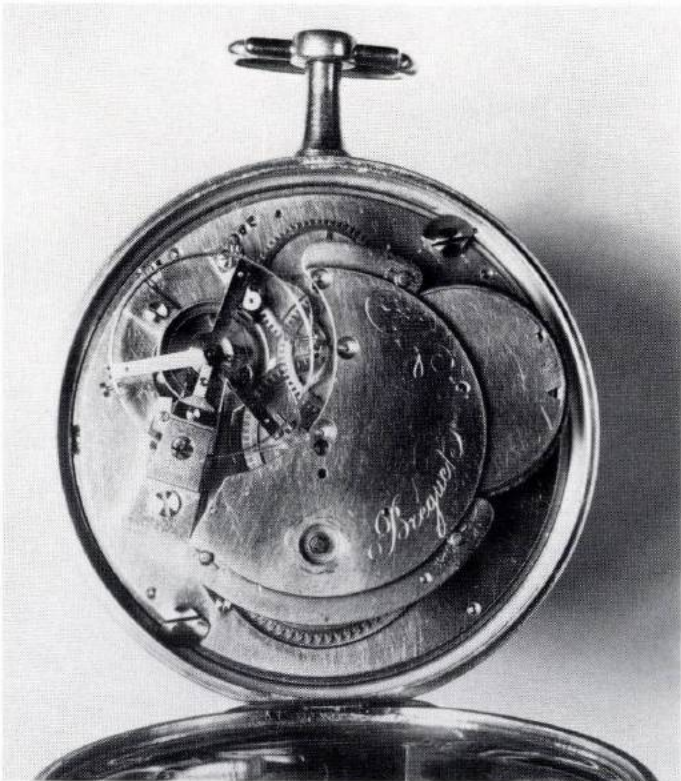
△ 14 Zertifikat für die Uhr von Abb. 11 und 12 15 Diese frühere Ausführung einer Taschenuhr mit Chronometerhemmung von A. L. Breguet mit der Nr. 147 hat die Räder noch nicht in Lochsteinen gelagert. Diese Grundkonstruktion wurde beibehalten. Sie hat Arnoldsche Federhemmung, dreiarmligen bimetallicischen Unruhreif, Wendelfeder, Parachute sowie Schnecke und Kette 15 ▽
