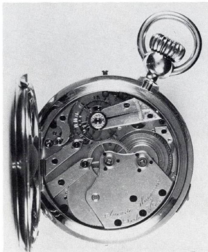
23 Schweizer Taschenuhr mit Wippen-Chronometerhemmung, signiert Huguenin, 2. Hälfte des 19. Jhs.
