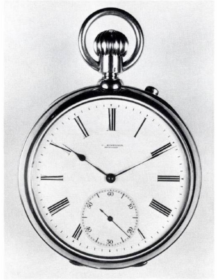
18 In der Schweiz hergestellte Taschenuhr mit Chronometerhemmung mit Feder nach Earnshaw. Die Signatur »C. Schweizer München« ist eine Händlersignatur
