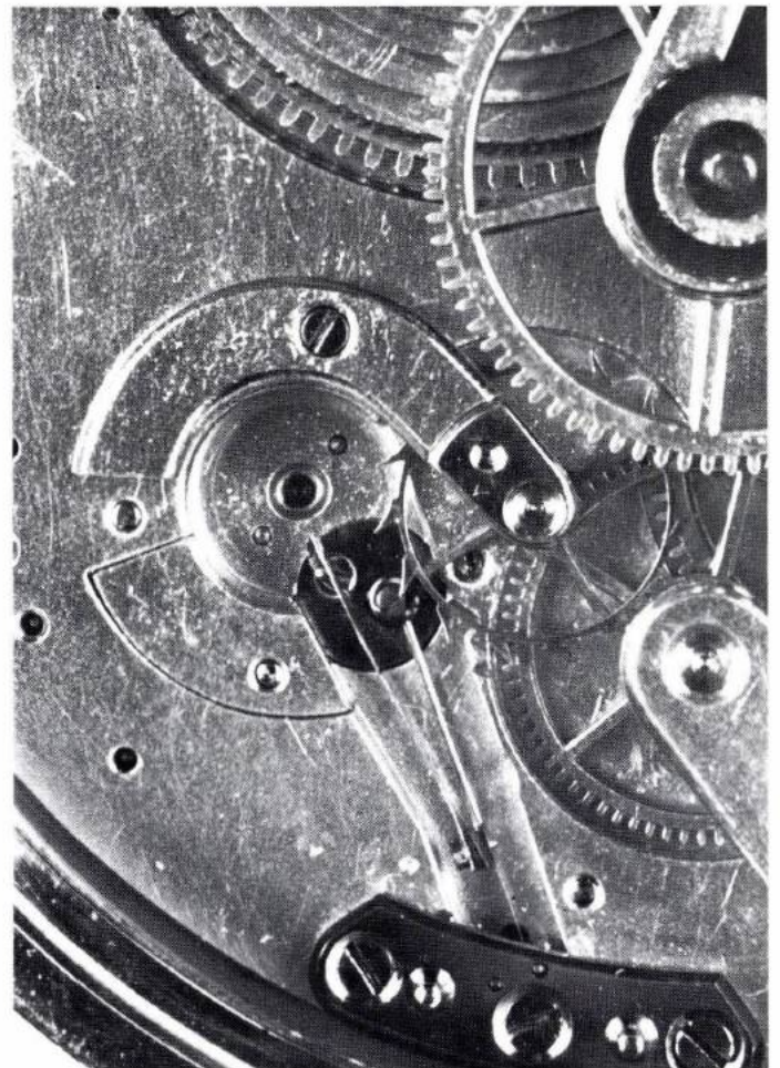
22 Die Chronometerfeder und Goldauslösefeder sowie Ruhestein und Steigrad nach Earnshaw der Uhr von Abb. 19
