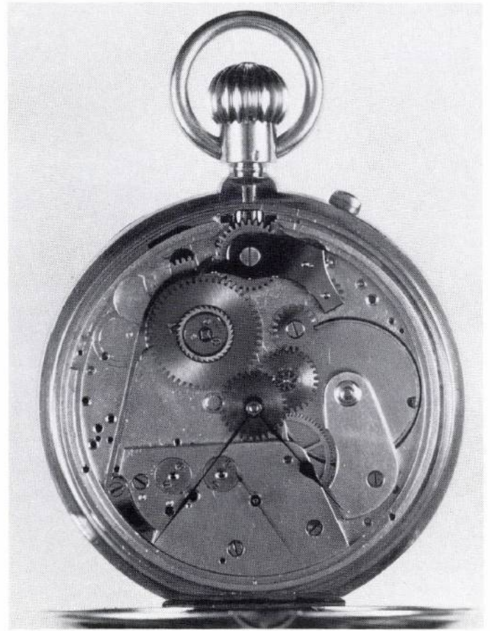
20 Beim Wippenaufzug der Uhr von Abb. 18 und 19 wird bei Friktionsbelastung eine Sperrklinke ausgelöst, die das Sperrrad auf dem Schneckenrad bewegt
