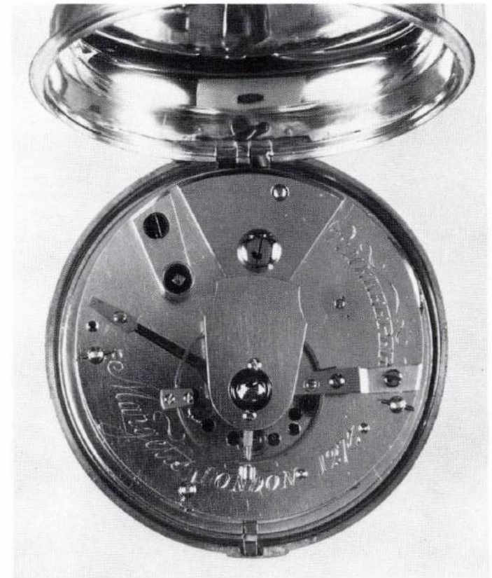
7 Taschenuhr mit Arnoldscher Chronometerhemmung, signiert Margetts London
