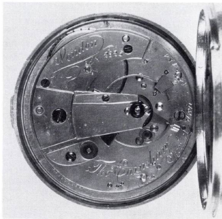
8 △ 8 Taschenuhr in Silbergehäuse mit Chronometerhemmung von Thomas Earnshaw, bei der ein einfacherer Unruhkloben vorhanden ist als bei Abb. 5
