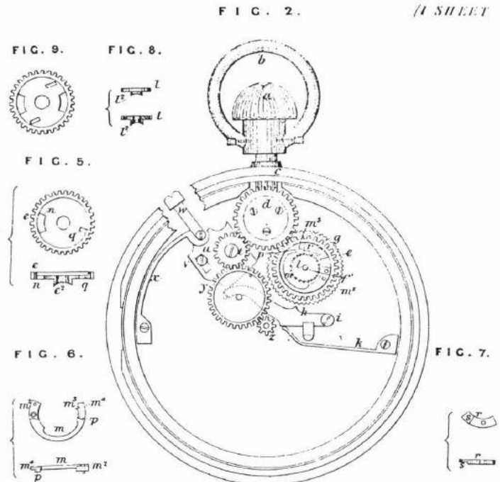
21 Patentschrift von 1864 von William Ehrhardt, die die eigenwillige Aufzugs-konstruktion der Uhr von Abb. 18, 19 und 20 zeigt
